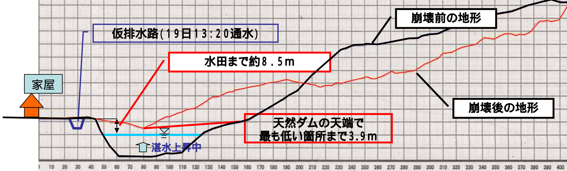
磐井川 市野々原地区 横断図 (水位は6月19日17時現在)
