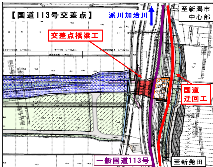
拡大平面図
