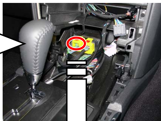
センタ・コンソール(パネルを外した状態)
