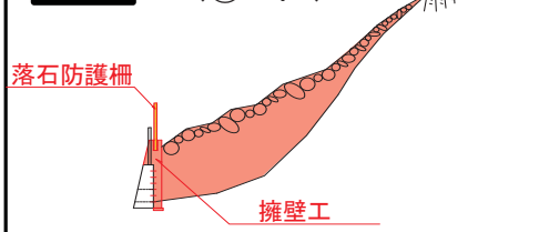
被害状況①工区
