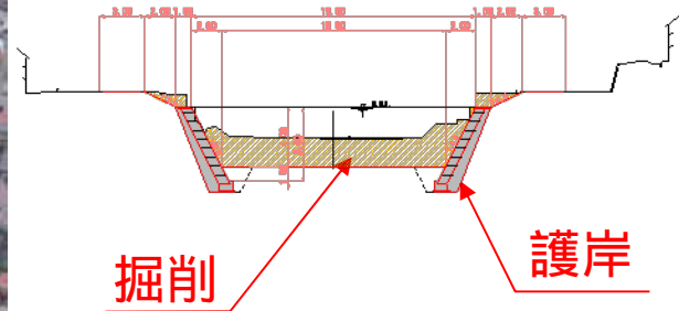
標準横断面図 (田川本川工区)
