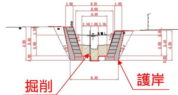
標準横断面図 (支川晒川工区)
