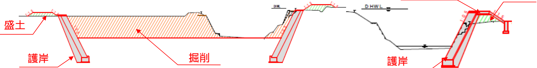
屈曲部対策（屈曲部是正、河道拡幅）
