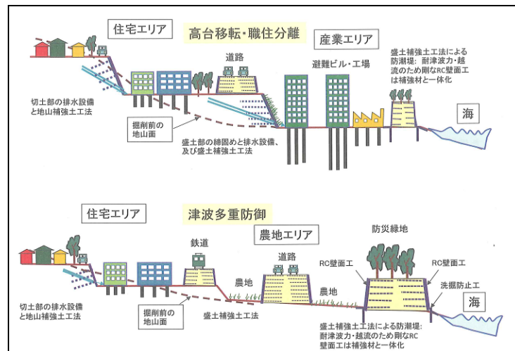
図17 多重津波防御施設と地盤工学的対応の例
