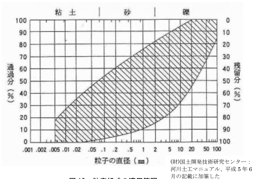
図 13 粒度組成の適用範囲
