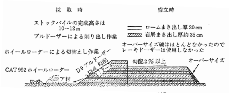
図 11 ストックパイルの例 (フィルダムの調査・設計から施工まで p. 264)
