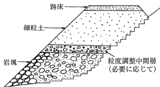
図1 粒度調整中間層の設置例（「道路土工 盛土工指針」p.168）
