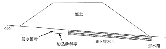
図9 湧水処理の例（道路土工 盛土工指針 p.171）
