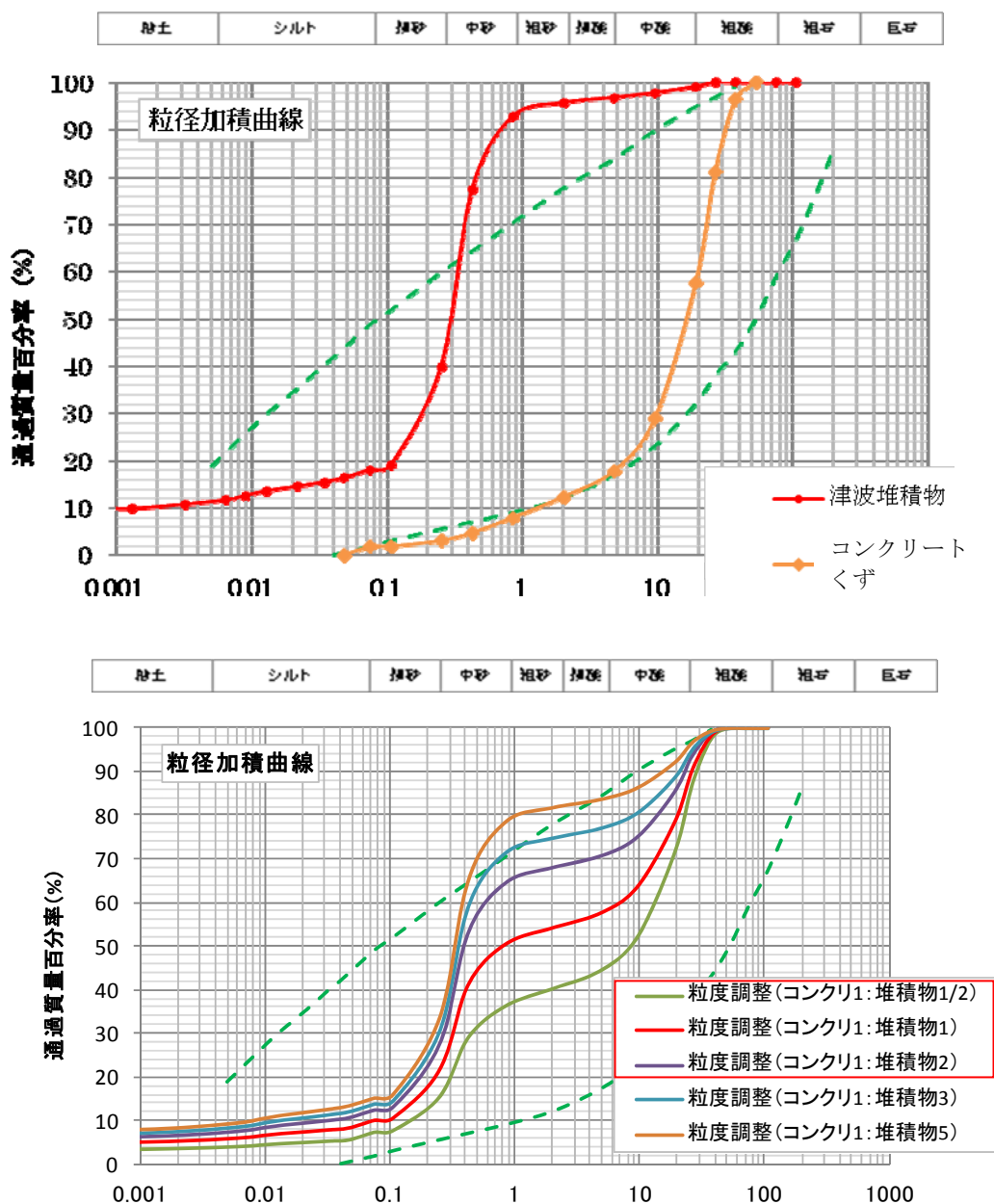
図 24 コンクリートくず及び津波堆積物の粒径加積曲線（上図） 両者の混合による粒度調整後の粒径加積曲線（下図）
