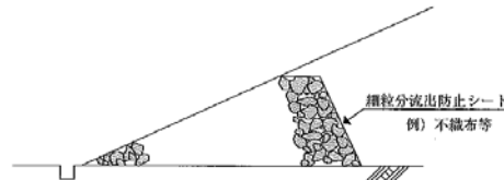
図4 のり尻工の例（道路土工 盛土工指針 p.158）
