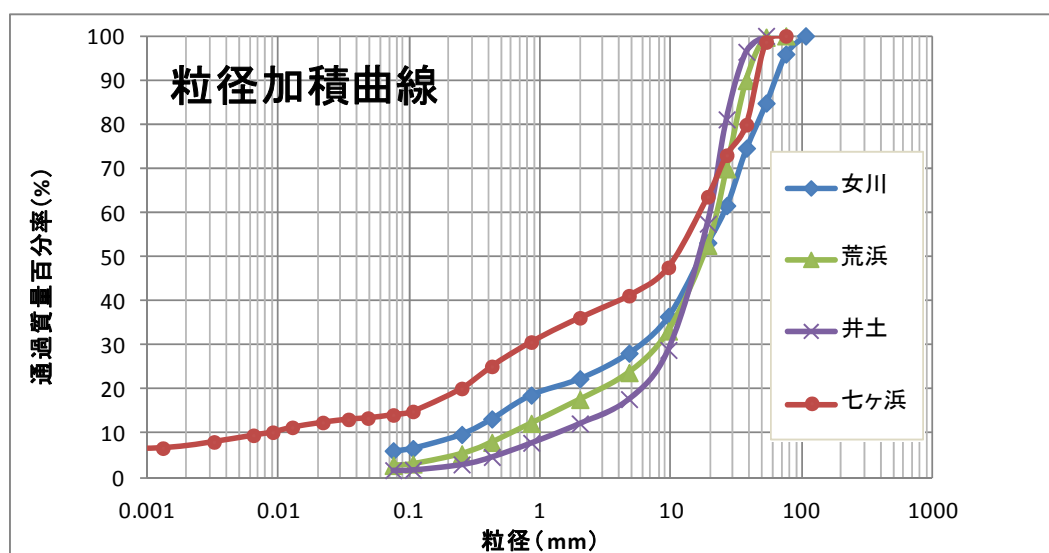
図20 コンクリートくずの粒径加積曲線
