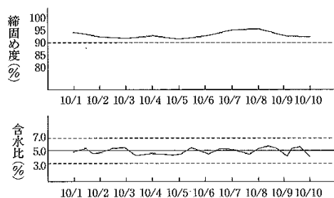
図14 \bar{x} \sim R 管理図の例
