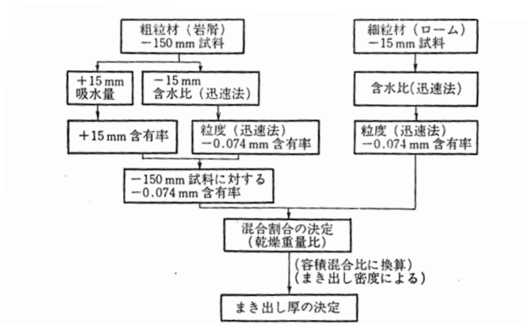
図 12 ストックパイルの品質管理フローチャートの例 (フィルダムの調査・設計から施工まで p. 264)
