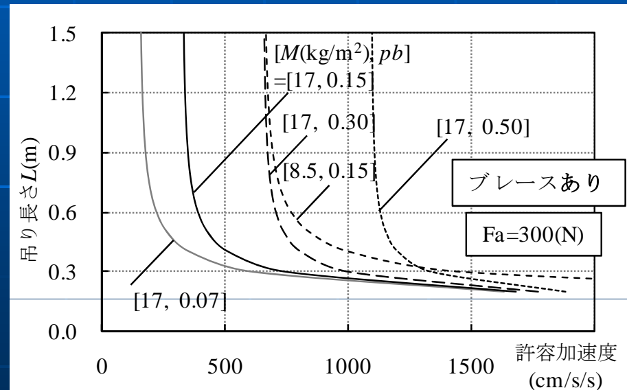
図 許容加速度
