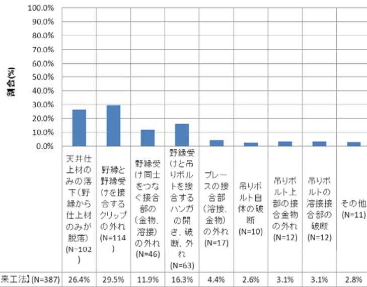
被害の概要【在来工法】(N=387)
