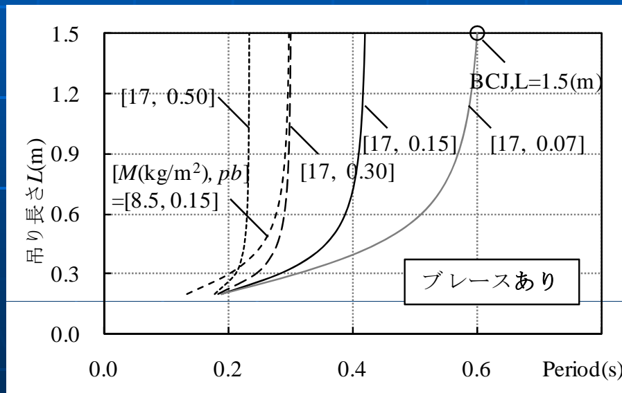
図 固有周期
