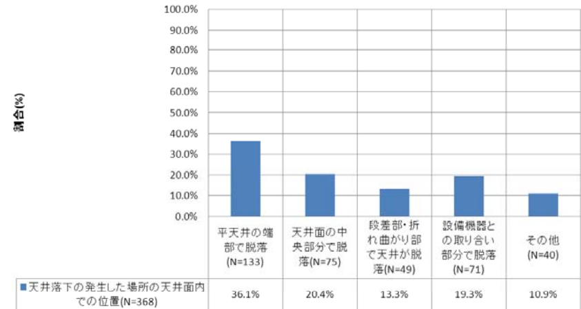
天井落下の発生した場所の天井面内での位置(N=368)
