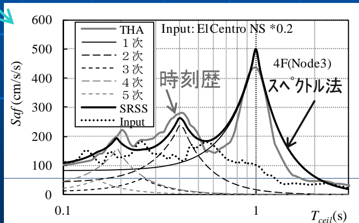
せん断型5階建て(5自由度系)の例
