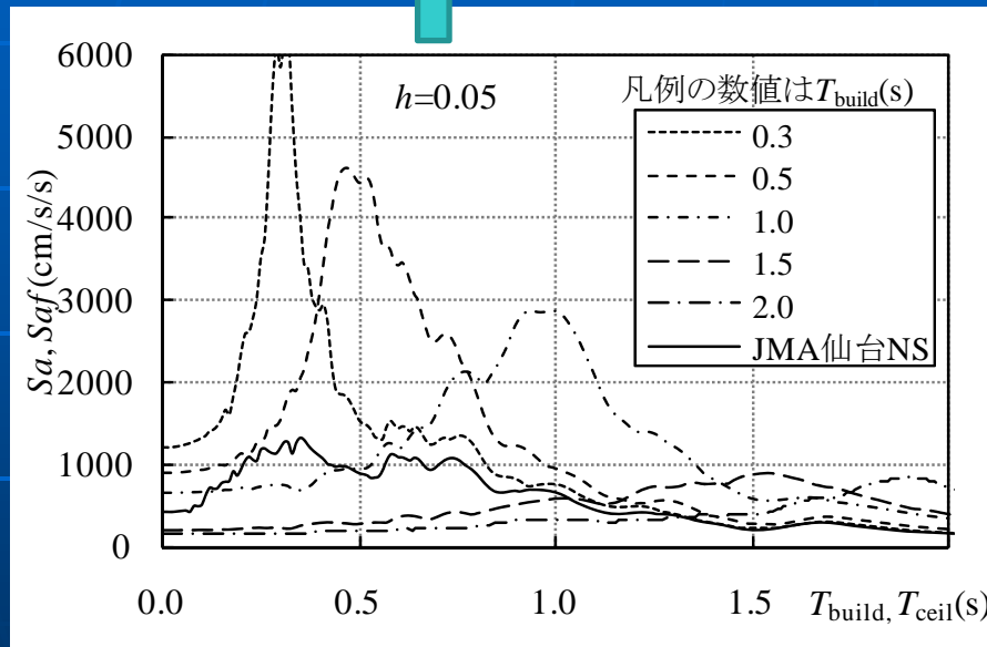
(a) S_a - T_{build} 関係 (実線) 及び S_{af} - T_{ceil} 関係 (点線等)
