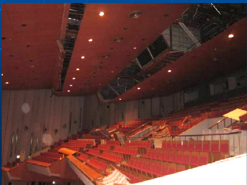
段差部・折り曲がり部
