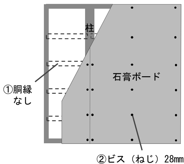
図1. 間仕切壁(イメージ)
