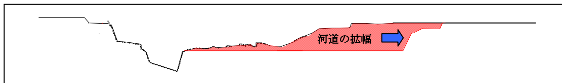
<星野川下流横断面図>
