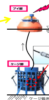
土研式水位観測ブイを設置(平成25年2月)
