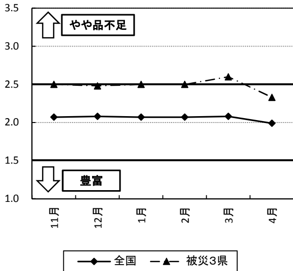
骨材(砂)
