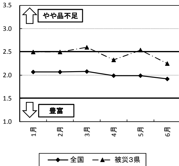
骨材(砂)
