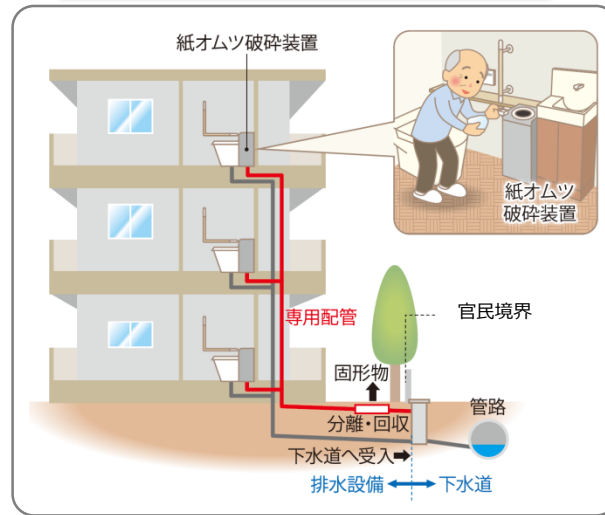
Bタイプ（破碎・回収タイプ）
