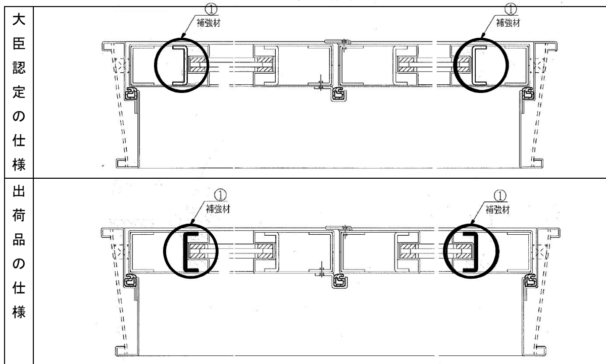
水平断面図
