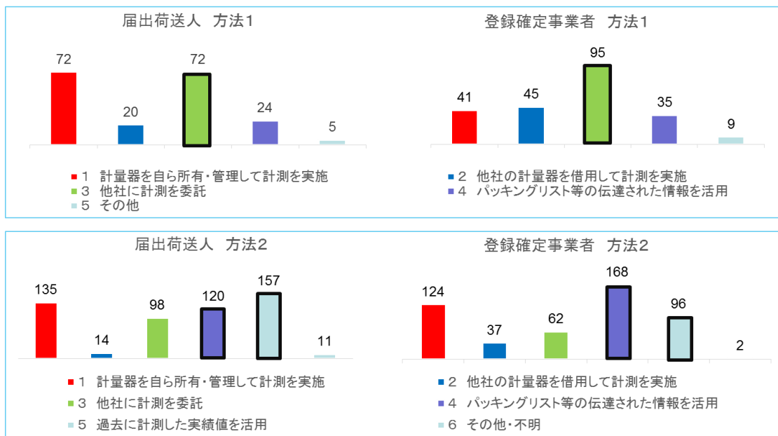
図9 コンテナ総重量の計測・算出方法
