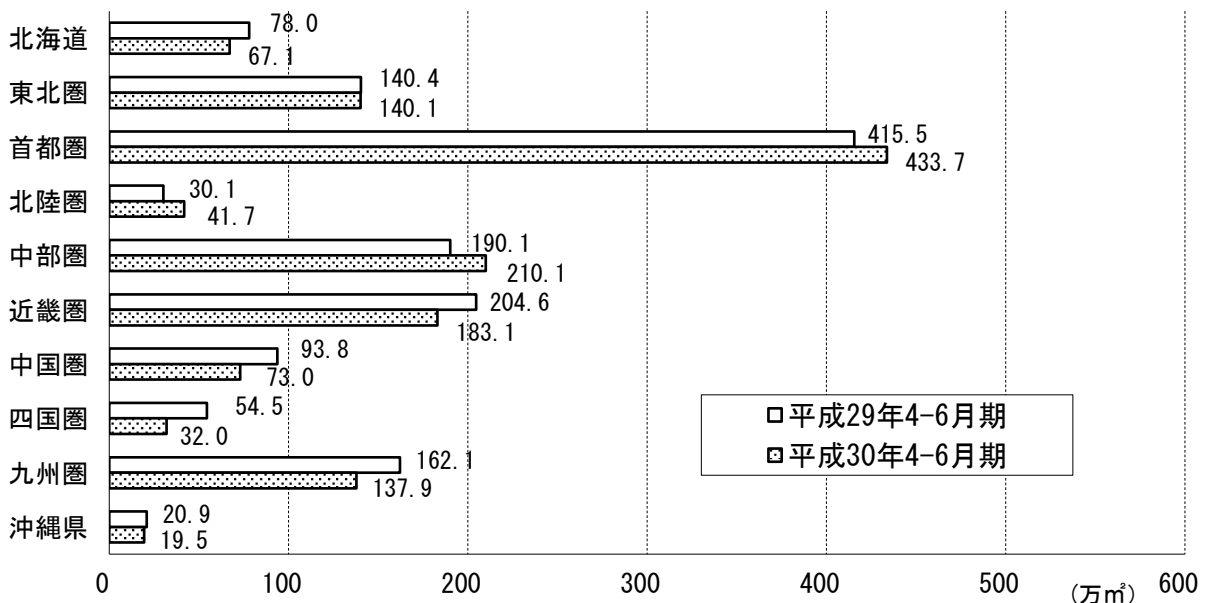
図 2-4-(3) 建築着工床面積(非居住用)(各広域ブロック、平成29年4-6月期、30年4-6月期)
