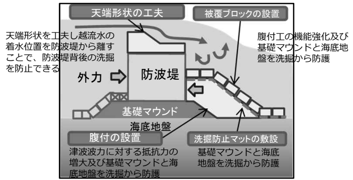
粘り強い構造とするための具体的な補強策
