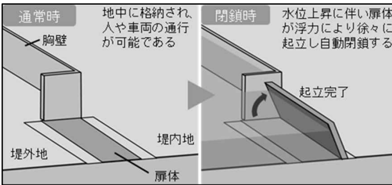
「津波による浮力で閉鎖」するフラップゲート式の陸閘の事例：撫養港海岸
