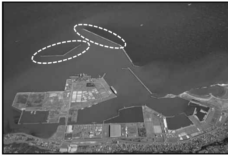
粘り強い構造の防波堤の整備事例：御前崎港
