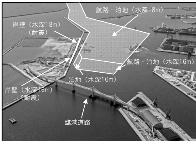
小名浜港の整備状況
