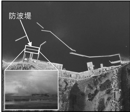
おくしり 奥尻港(奥尻島)における整備事例
