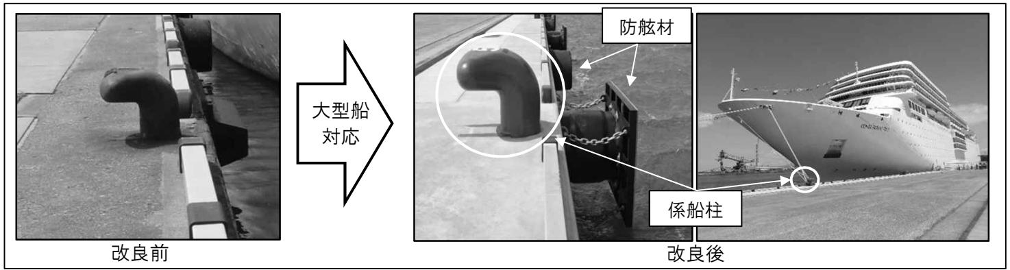
既存ストックを活用したクルーズ船の受入れ：酒田港
