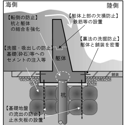
粘り強い構造の胸壁のイメージ
